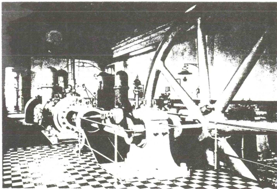
De „Jaffa“-machine, 1902
